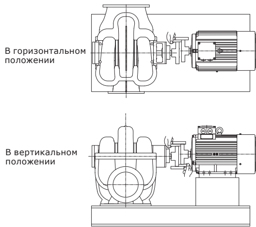
Рис. 37 Проверка соосности
