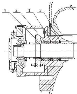
Рис. 12 Подшипниковый узел с сальниковой бужа
