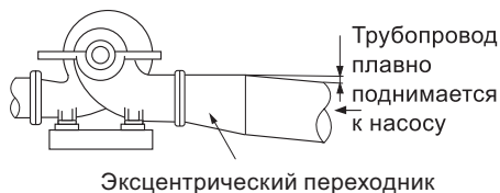
Рис. 29 Правильно смонтированный всасывающий трубопровод
