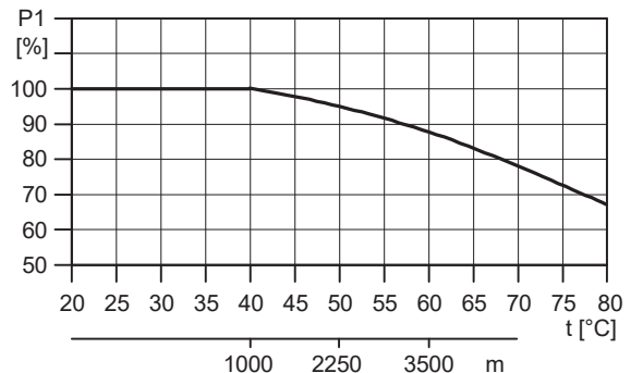
Рис. 40 Соотношение между мощностью двигателя (P2) и температурой окружающей среды (P1)
