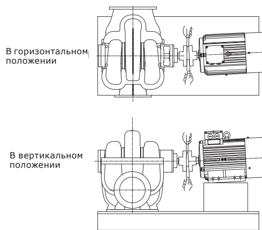
Рис. 36 Проверка углового выравнивания
