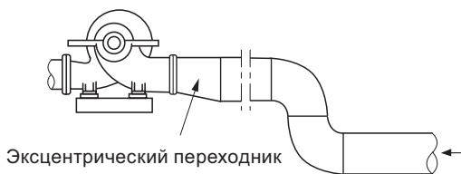
Рис. 31 Правильно смонтированный всасывающий трубопровод
