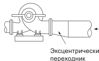
Рис. 26 Правильно смонтированный переходник
