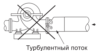
Рис. 27 Переходники, из-за которых образуются воздушные пробки и турбулентность
